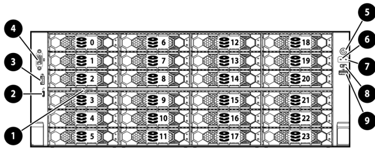
图1 前面板-24LFF 硬盘
