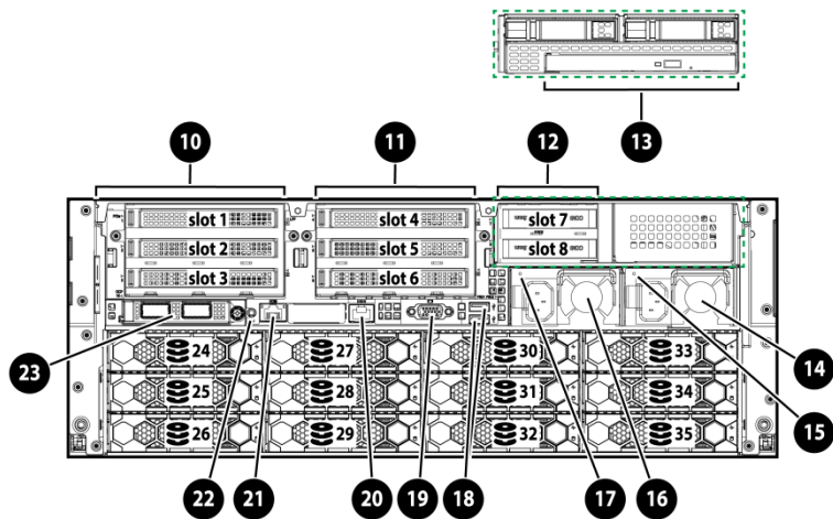
图2 后面板
