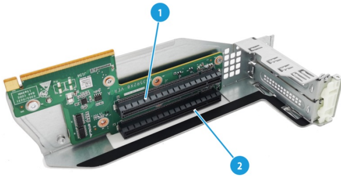
图10 RC-2HHHL-R3-2U-G5
