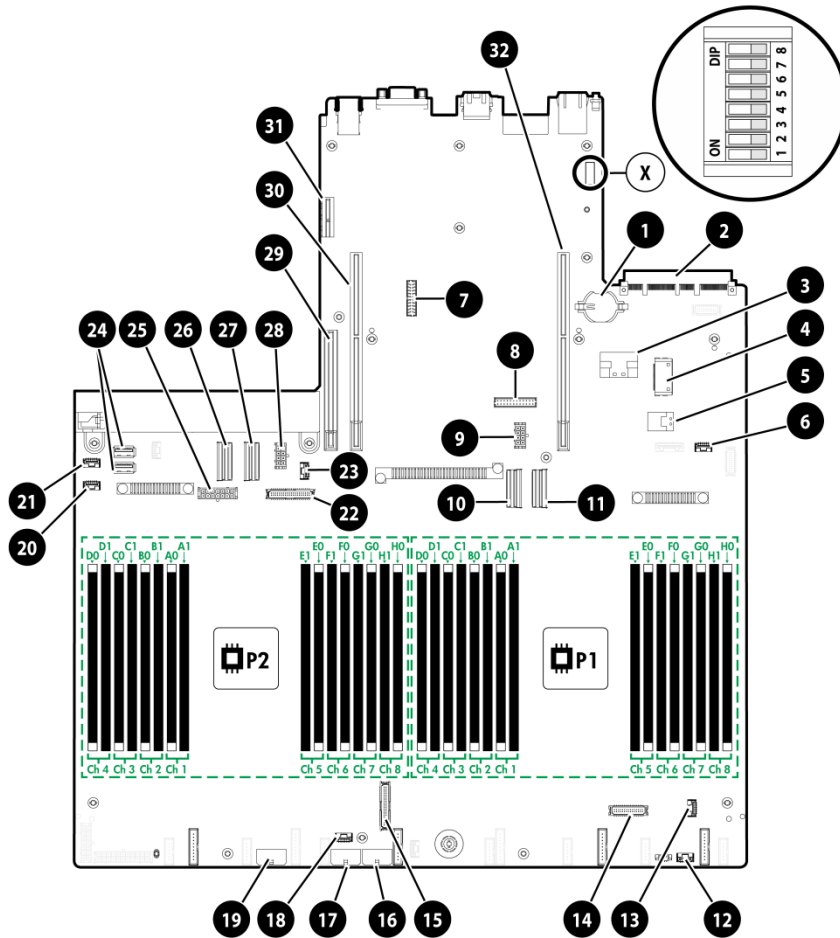
图5 R3630 G5 主板组件图
