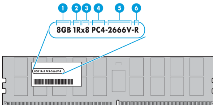
图12 内存标识
